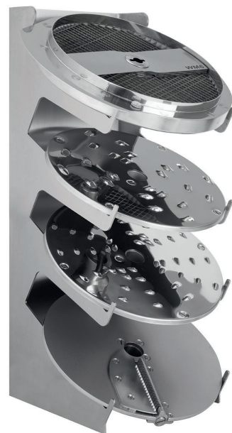
Scheibenstände für 4 oder 6 Scheiben liegend und stehend
