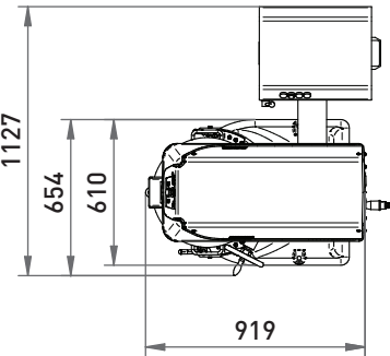
Maschine ohne Ansteckapparat
