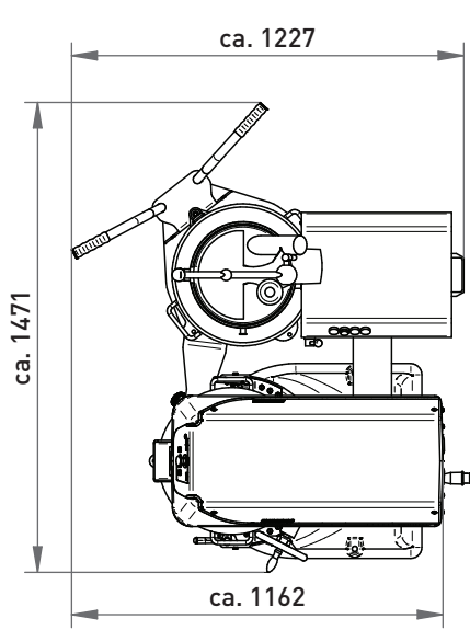
Maschine mit Ansteckapparat und Kesselwagen
