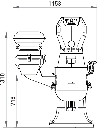
Maschine mit Ansteckapparat
